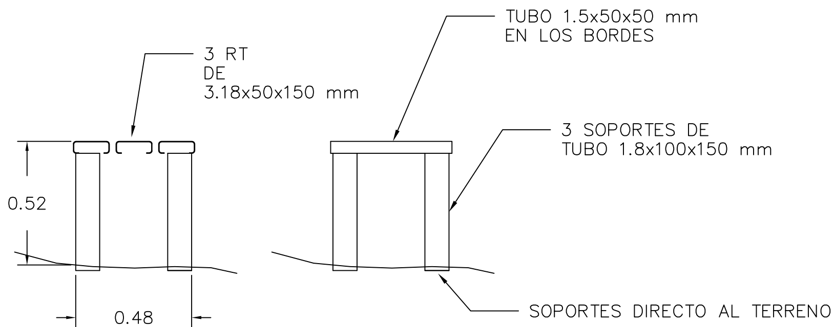
DETALLE DE BANCA EXISTENTE CANCHA ESTE (DOS UNDADES)
