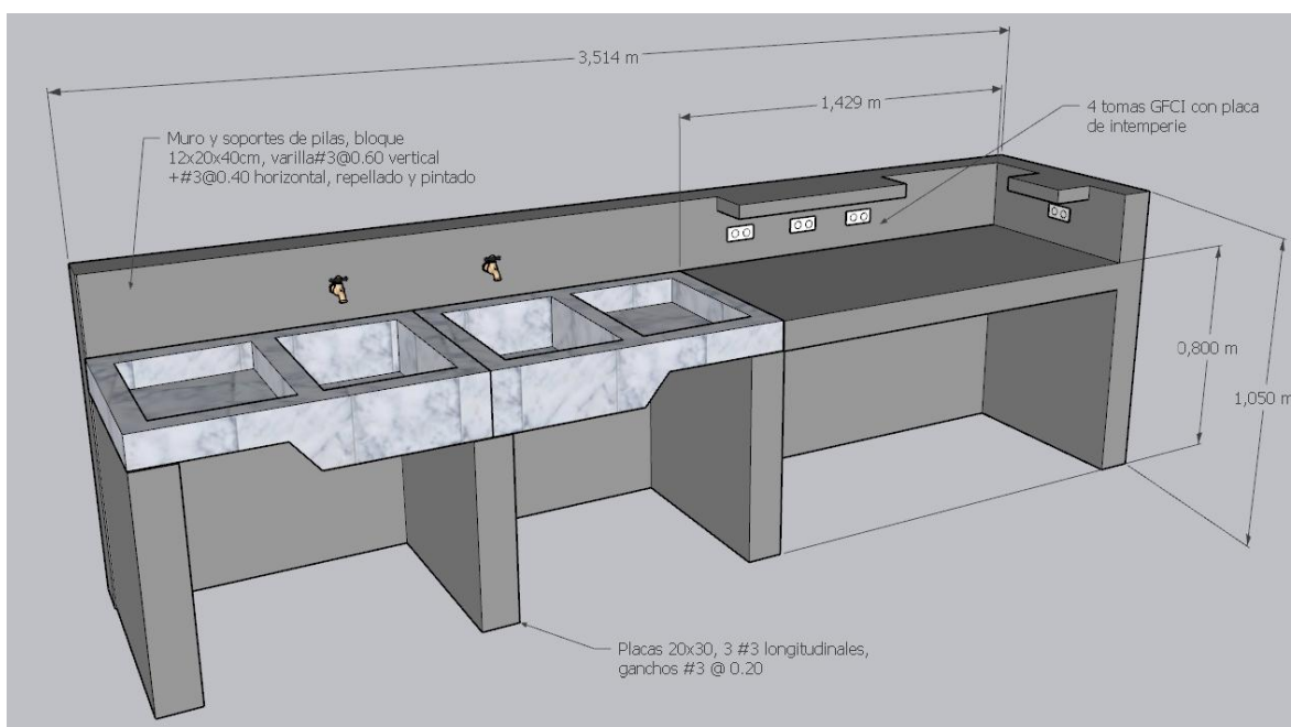
DETALLE DE LAS PILAS DE LAVADO
