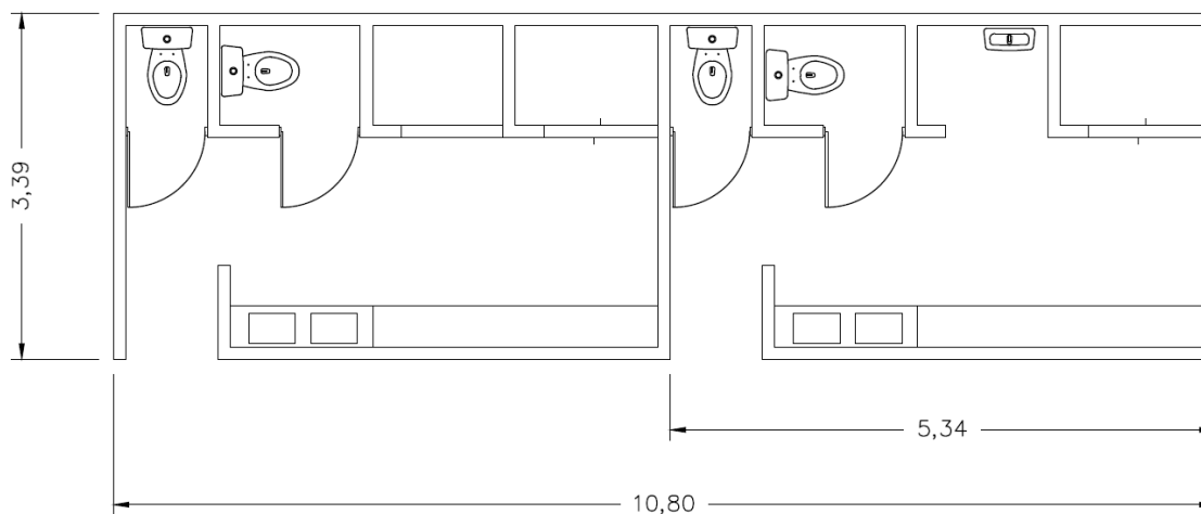
PLANTA SERVICIOS SANITARIOS EXISTENTES
