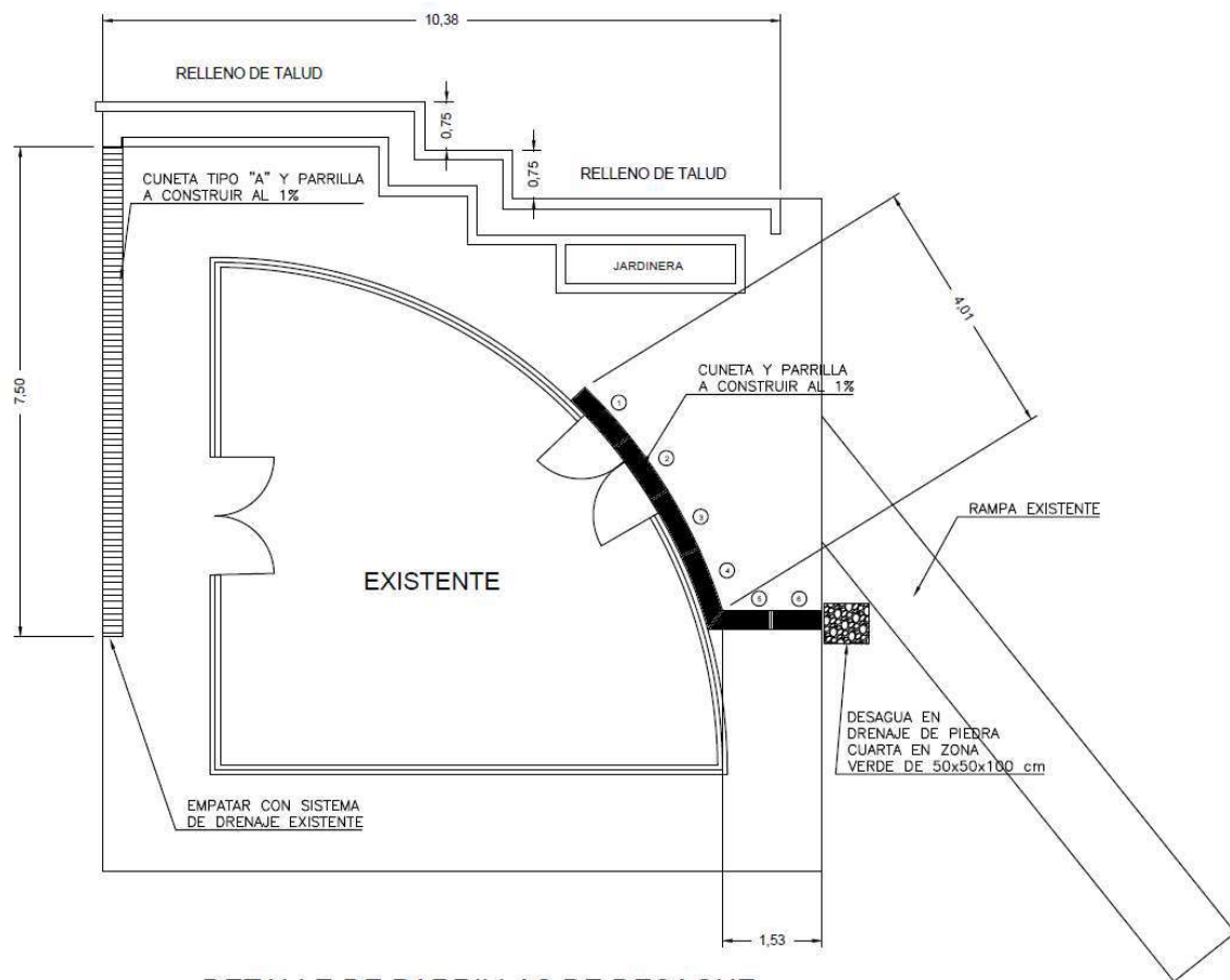
DETALLE DE PARRILLAS DE DESAGUE
