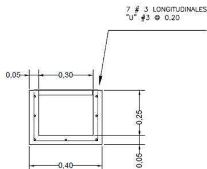
CUNETA TIPO "A"
