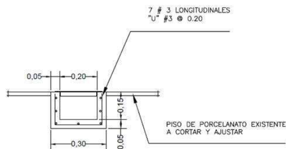
CUNETA TIPO "B"
