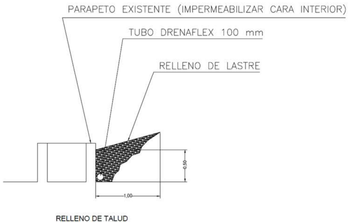
Imagen 4. Detalle relleno
