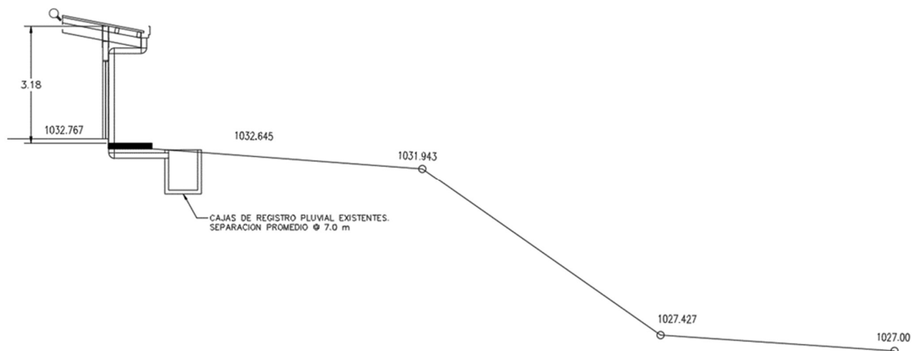
SECCION TIPICA EXISTENTE
