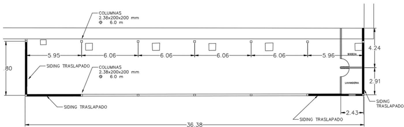
PLANTA ARQUITECTONICA
