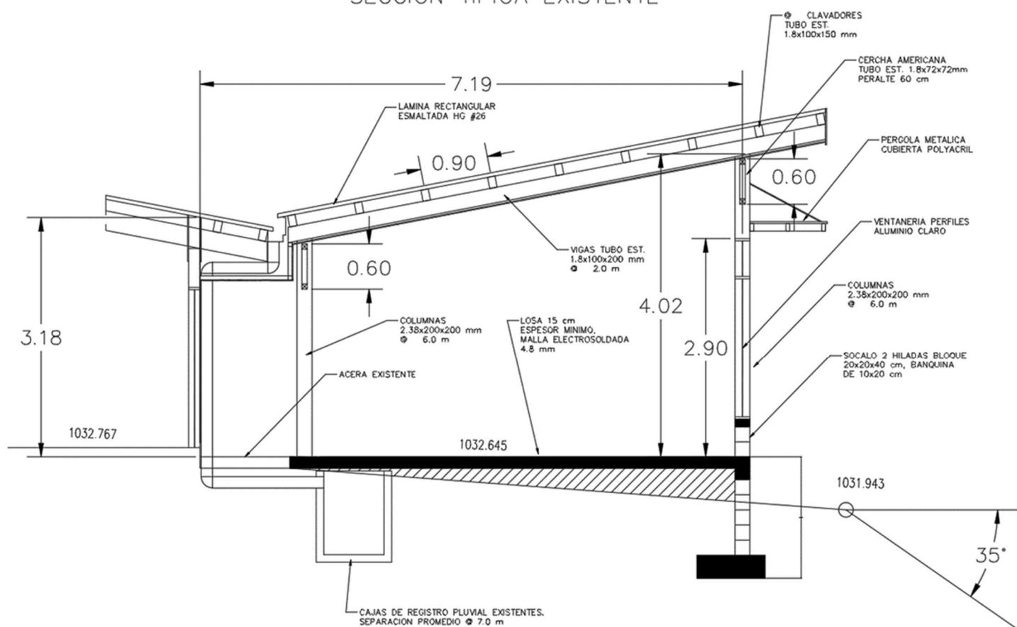
SECCION TIPICA EXISTENTE
