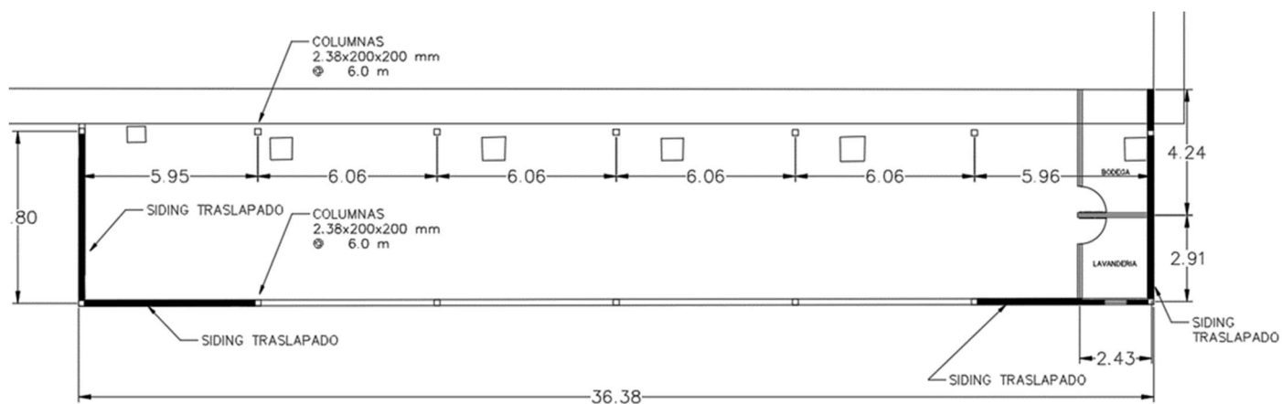
PLANTA ARQUITECTONICA
