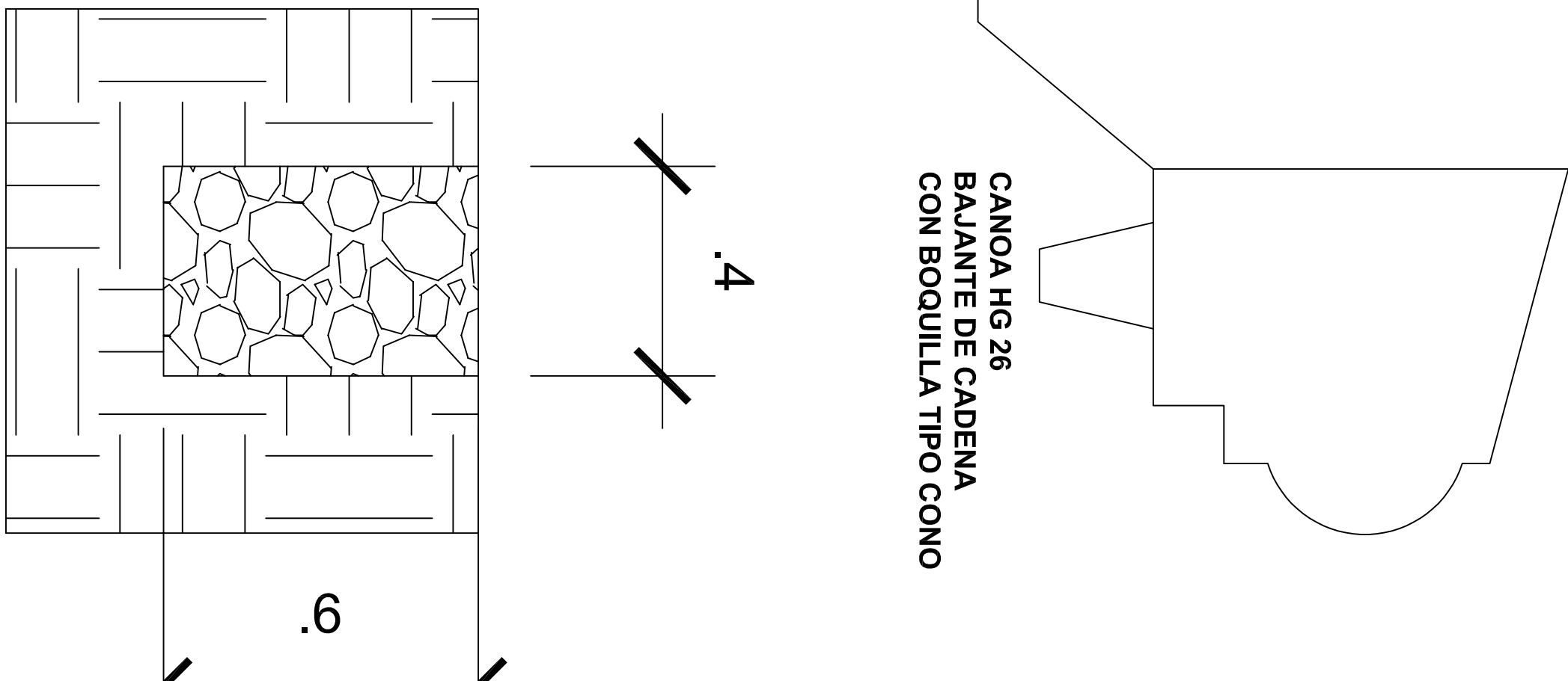
DETALLE CAÑO
