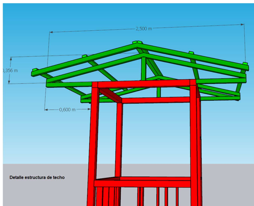
Imagen 10. Estructura de techo caseta de seguridad.
