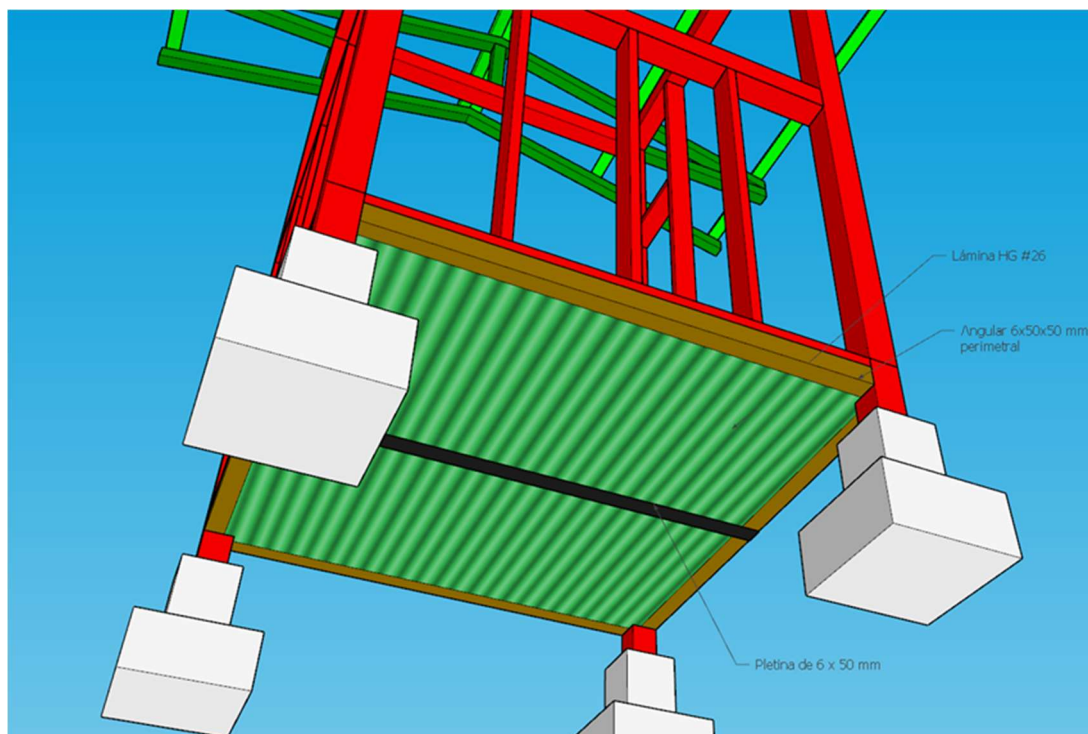
Imagen 7. Estructura caseta de seguridad.
