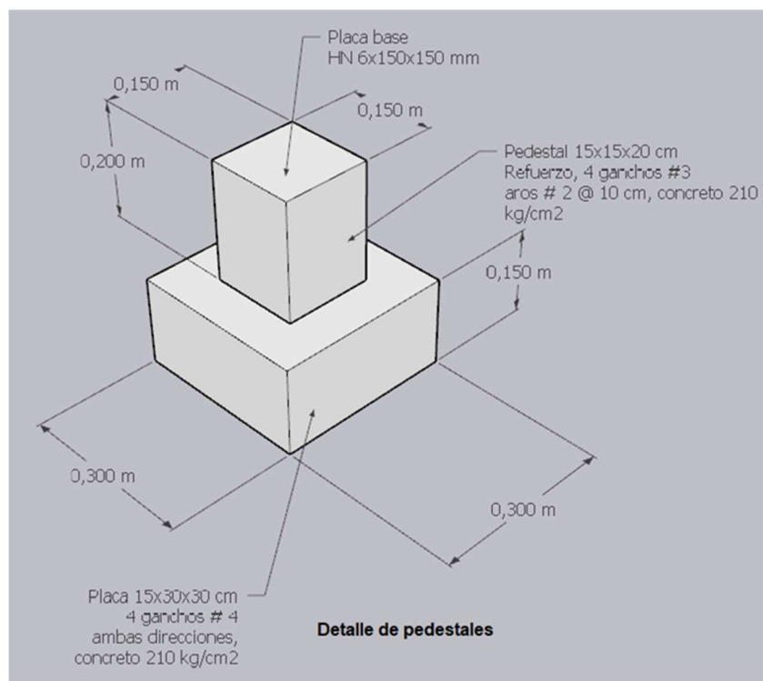
Imagen 8. Detalle de pedestal caseta de seguridad.
