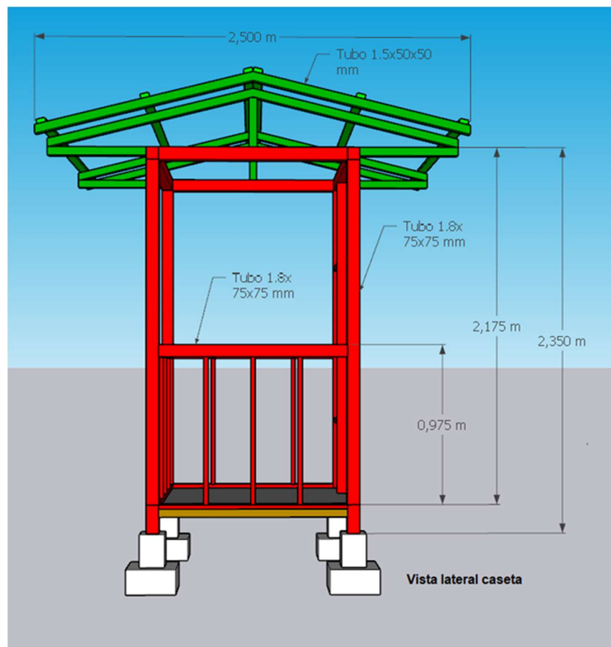
Imagen 6. Estructura caseta de seguridad.
