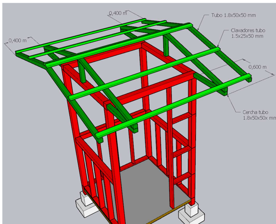
Imagen 9. Estructura de techo caseta de seguridad.
