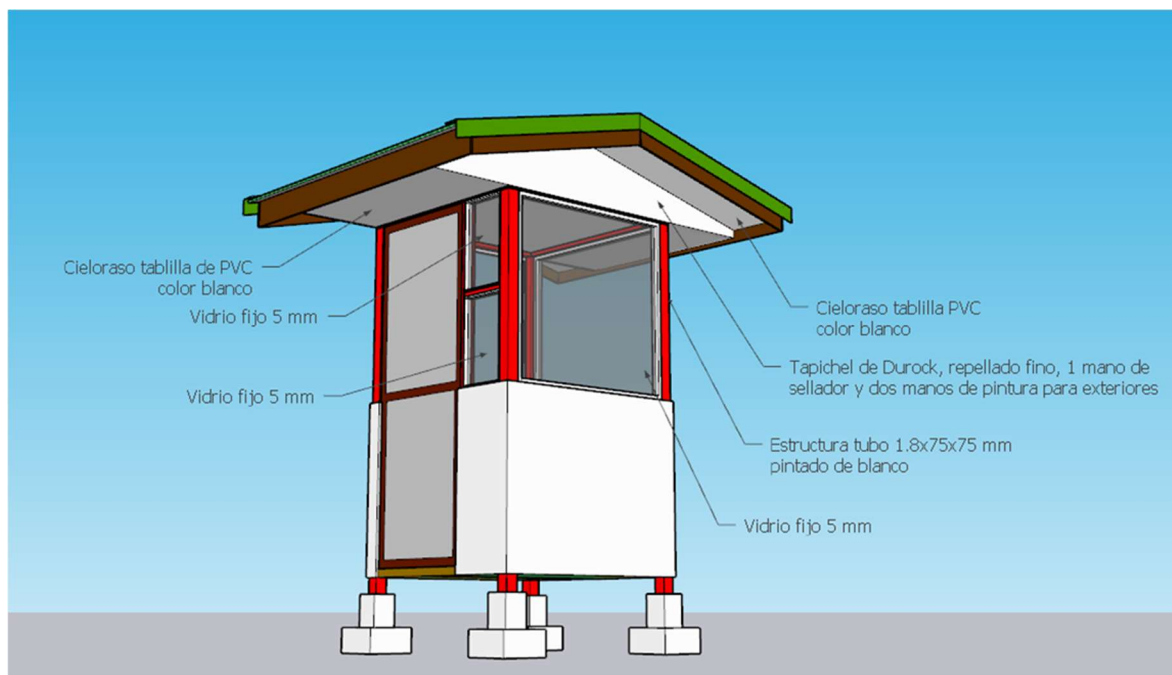
Imagen 11. Caseta de seguridad.
