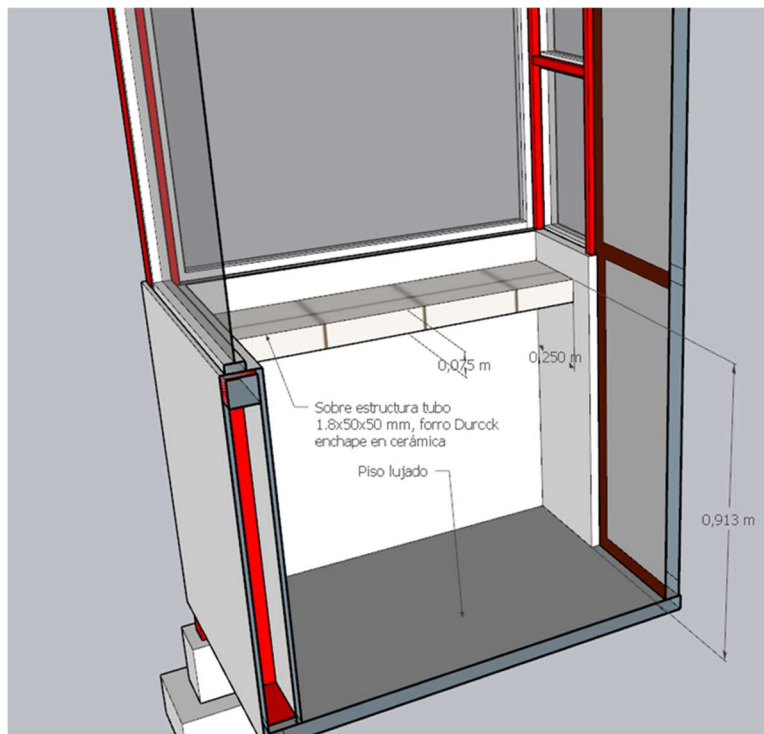
Imagen 13. Caseta de seguridad.
