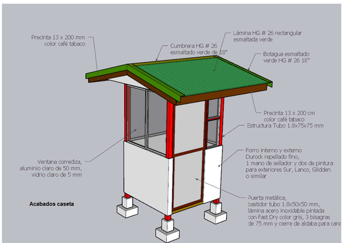
Imagen 12. Caseta de seguridad.
