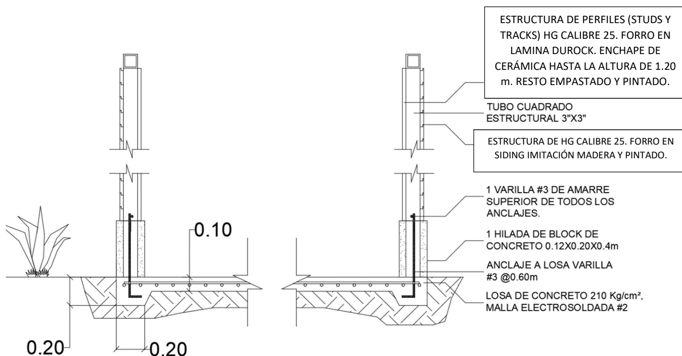
Imagen 13. Detalle vista lateral servicios sanitarios.
