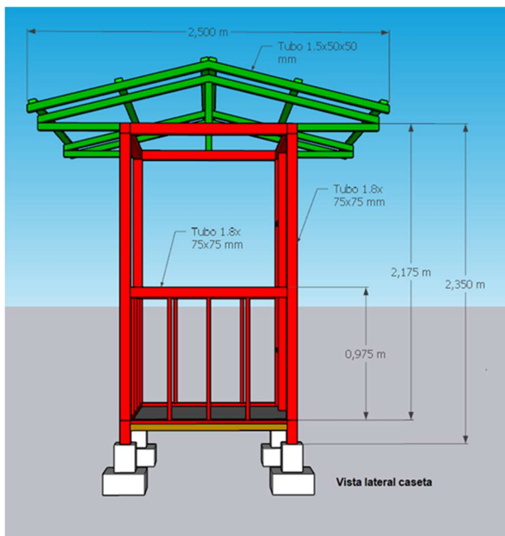
Imagen 20. Detalle estructural 2.
