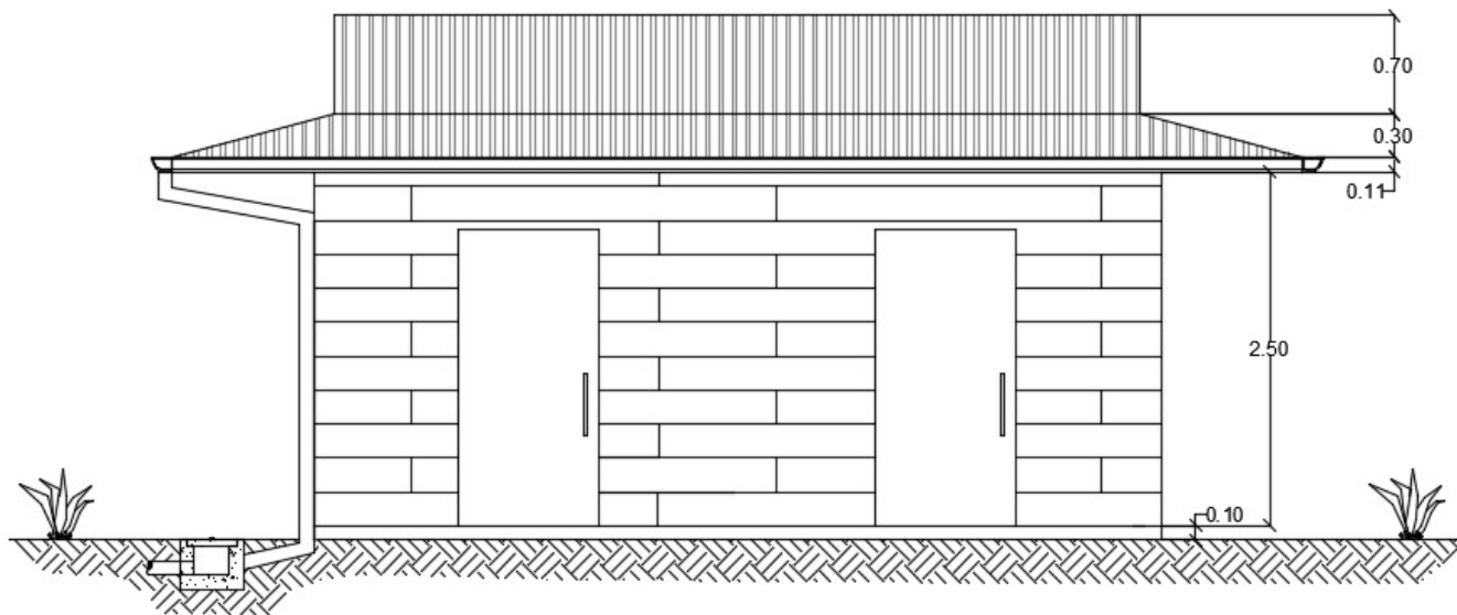
Imagen 11. Detalle vista frontal servicios sanitarios.
