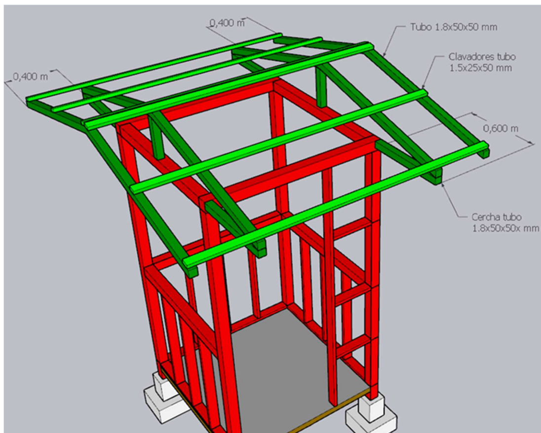
Imagen 23. Detalle estructura de techo.
