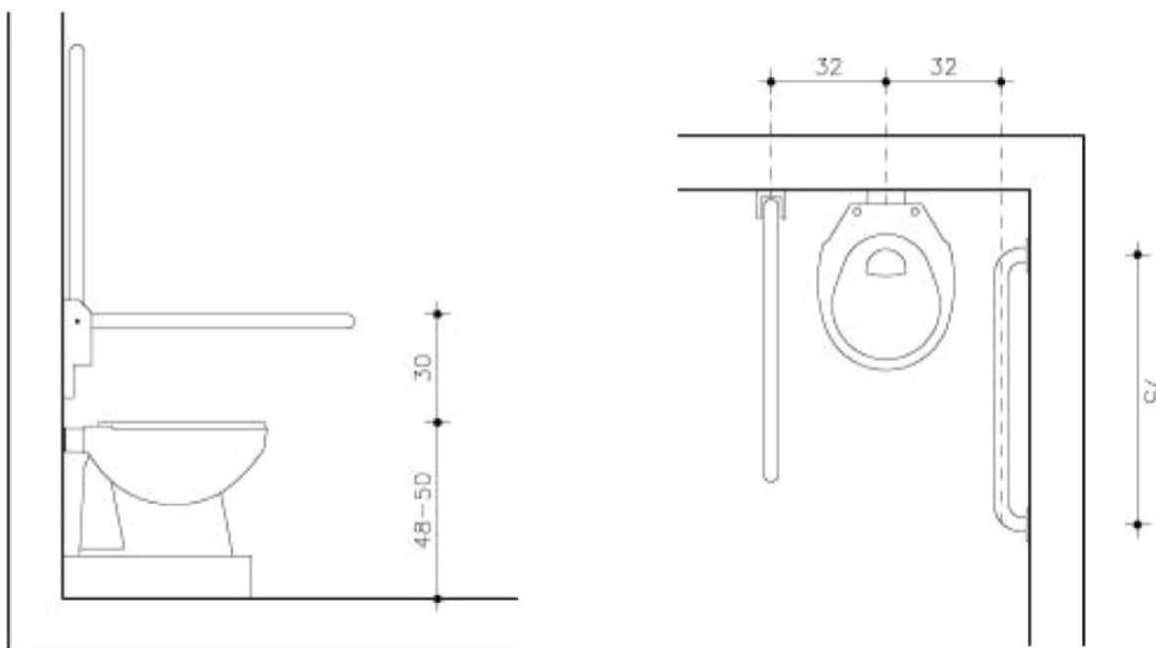
Imágenes 16. Inodoros Ley 7600.
