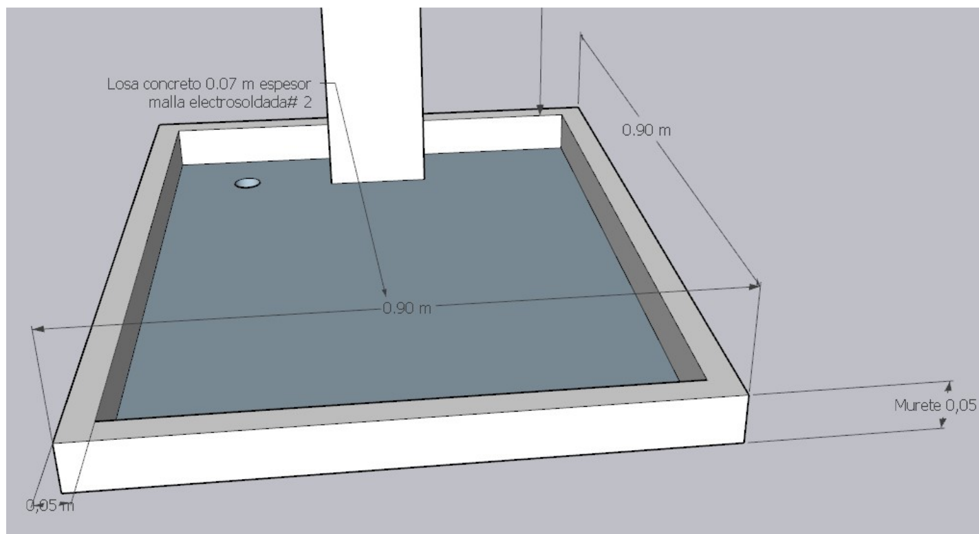
Imagen 8. Detalle de losa de ducha 1.
