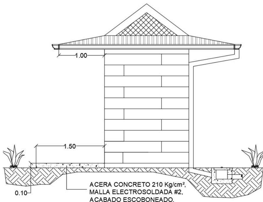
Imagen 13. Detalle vista lateral servicios sanitarios.
