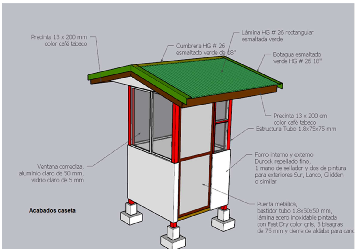
Imagen 26. Detalle acabados caseta.
