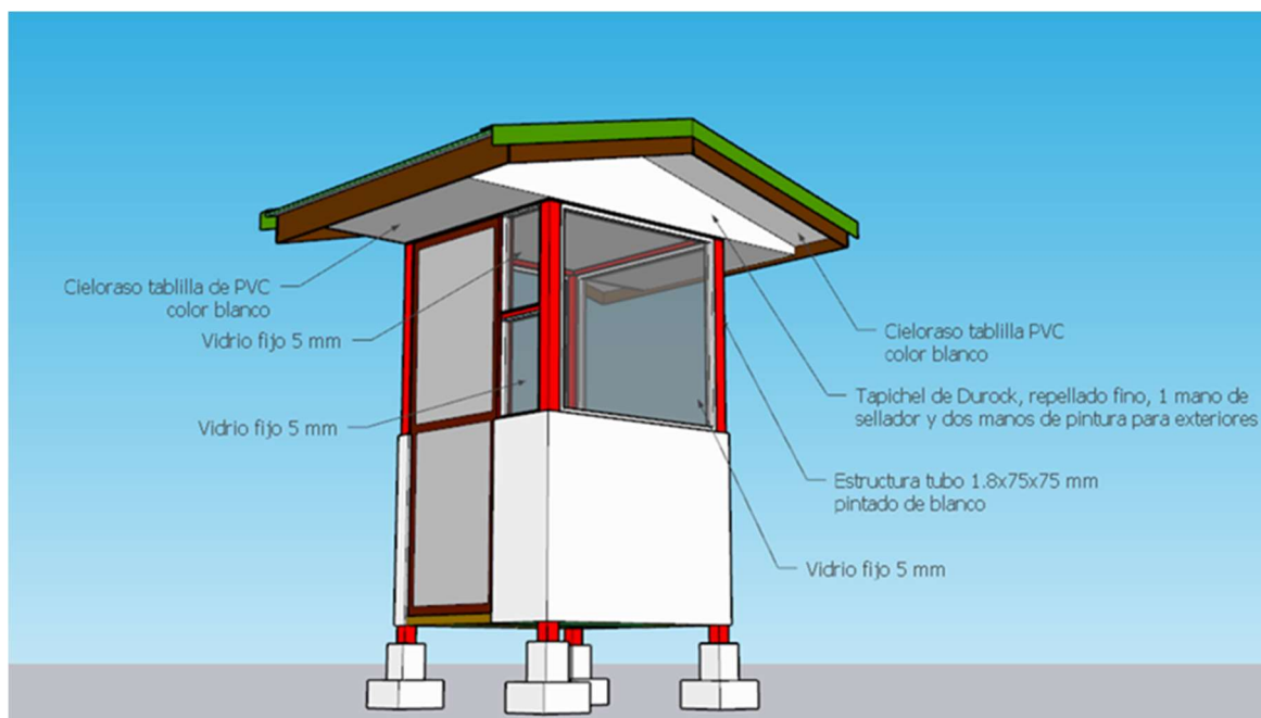
Imagen 25. Detalle caseta 1.
