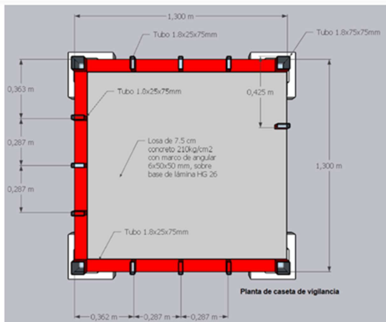
Imagen 18. Planta de caseta.
