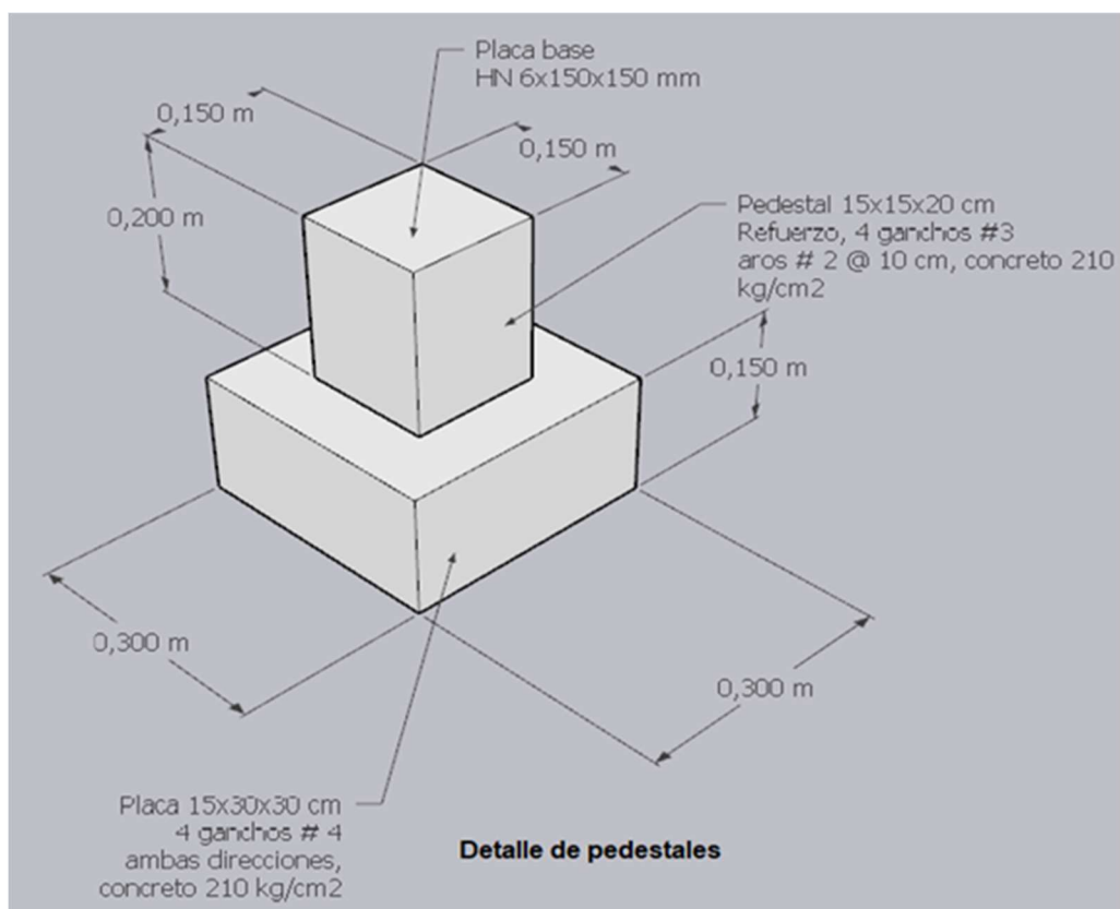
Imagen22. Detalle de pedestales.
