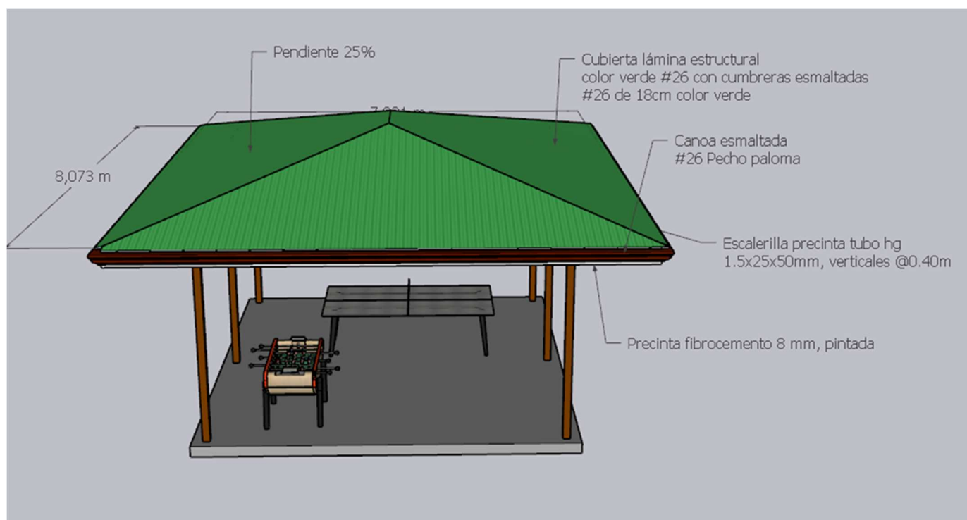
Imagen 2. [MQE2] Estructura y vigas.
