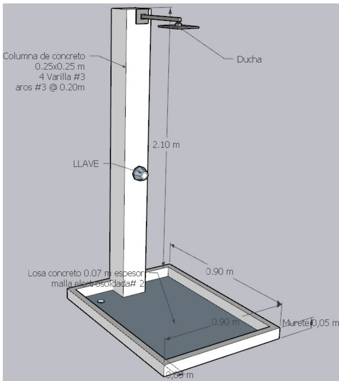
Imagen 7. Detalle de ducha 1.
