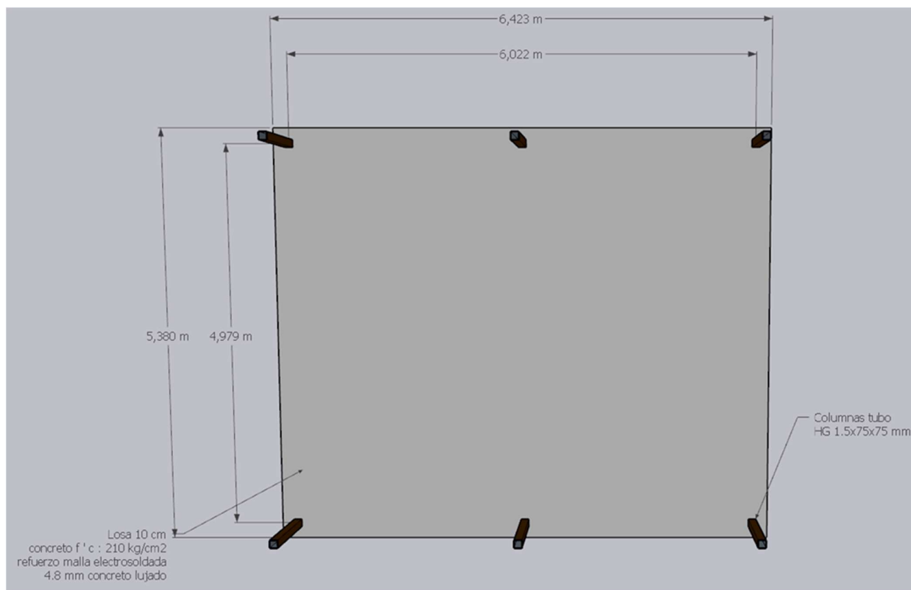
Imagen 1. Planta de rancho.
