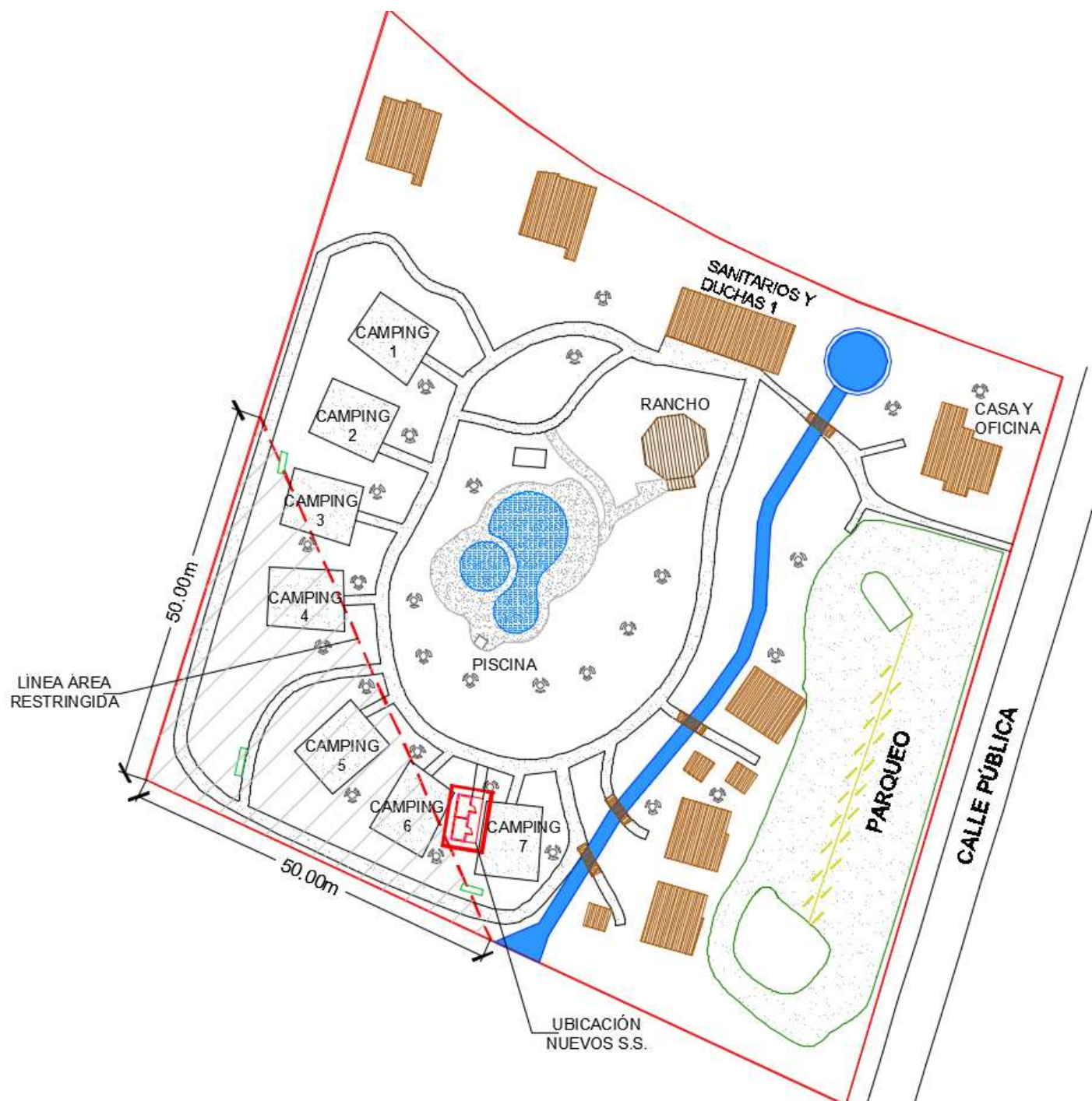
Imagen 15. Ubicación de nuevos servicios sanitarios dentro del Centro de Recreo.
