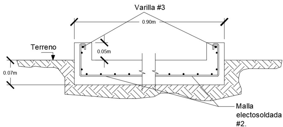
Imagen 9. Detalle de losa y murete de ducha.
