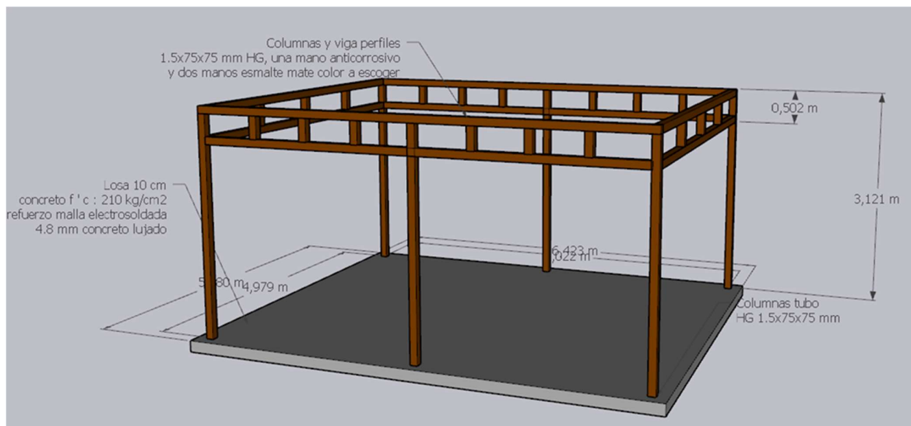
Imagen 2. [MQE2] Estructura y vigas.
