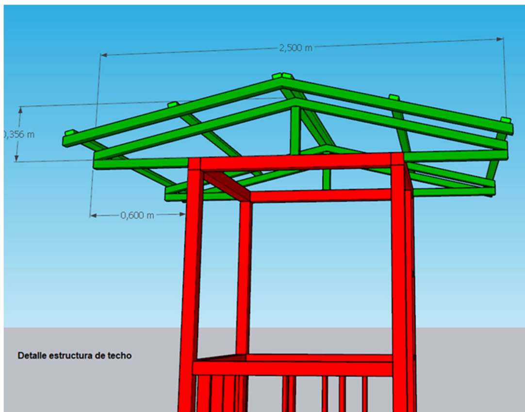
Imagen 24. Detalle estructura de techo.
