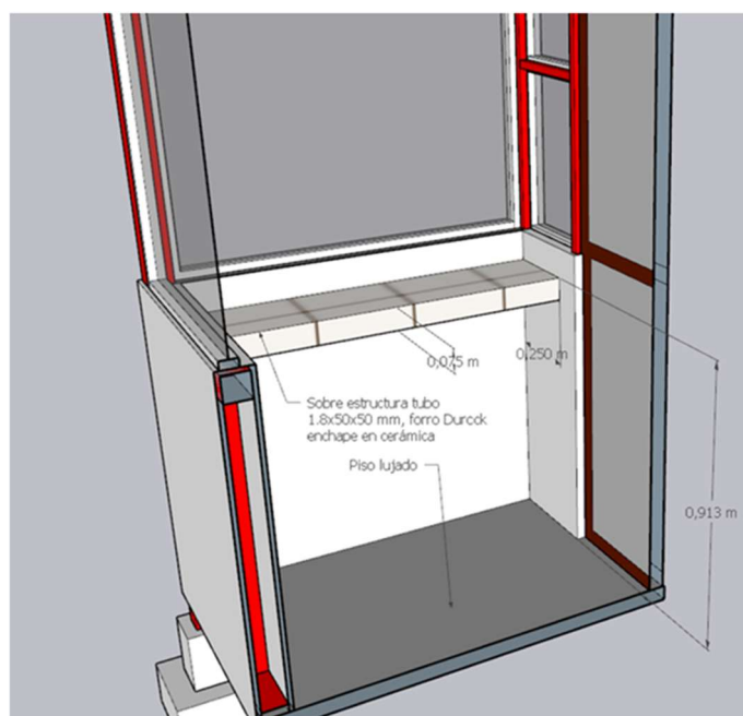
Imagen 27. Detalle acabados caseta 2.
