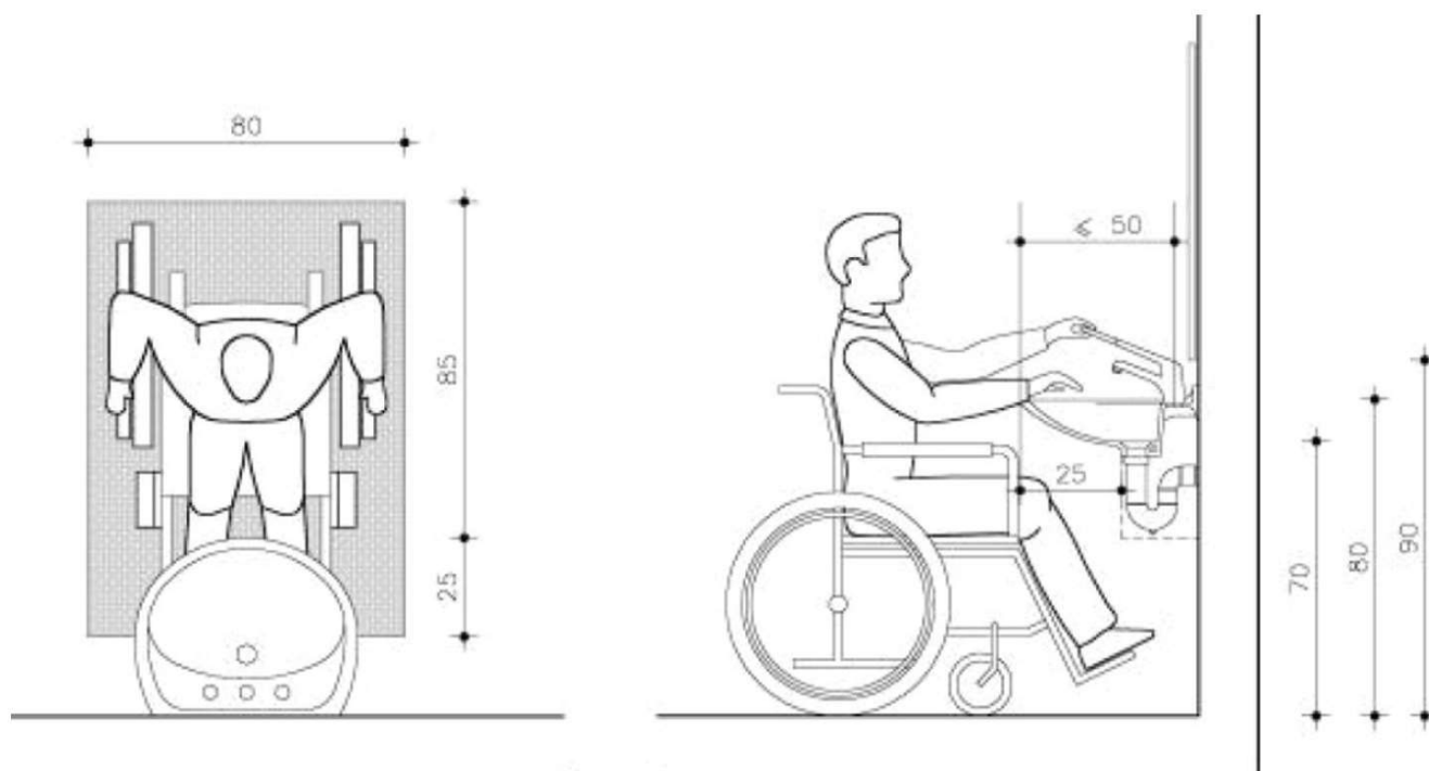
imágenes 17. Lavatorios Ley 7600.
