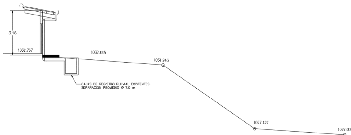
SECCION TIPICA EXISTENTE
