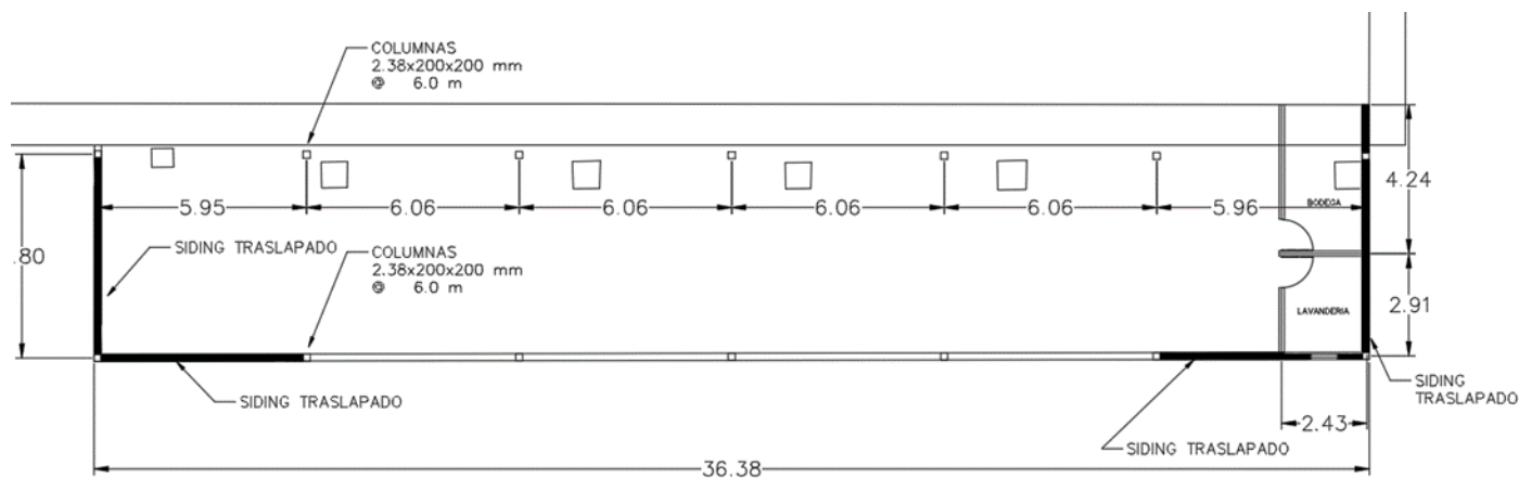
PLANTA ARQUITECTONICA
