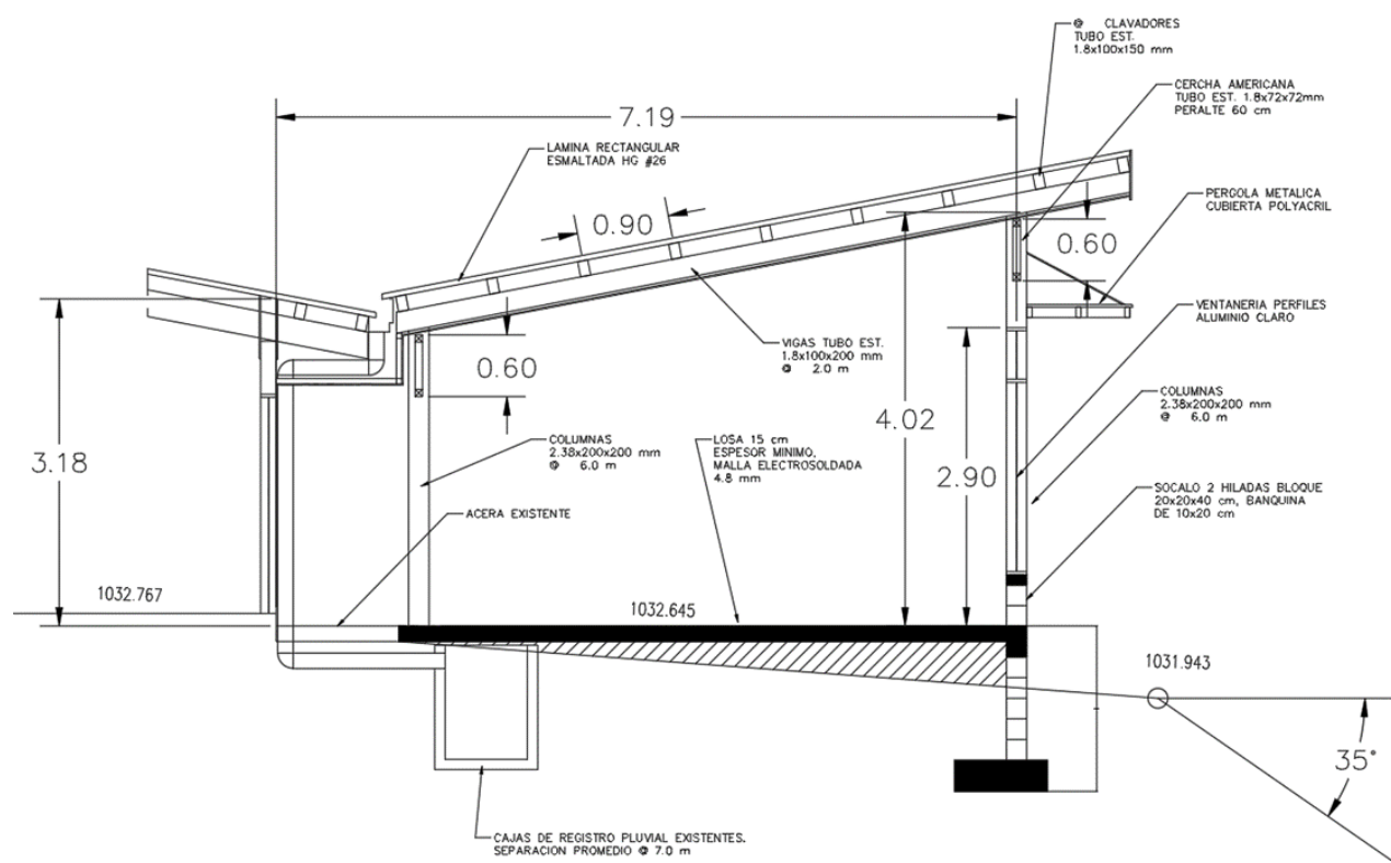
SECCION TIPICA PROPUESTA
